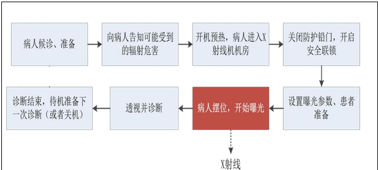
图 9-3 ERCP 专用 X 线成像系统操作流程及产污环节示意图
